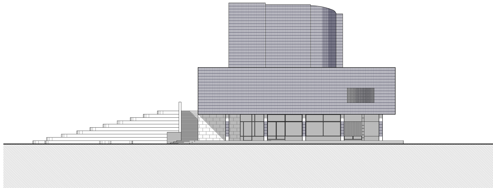
Alçat est
