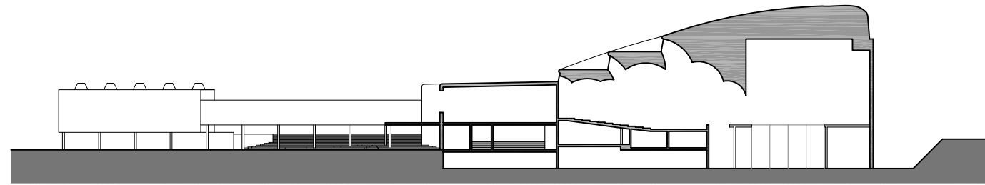
Secció B-B'
