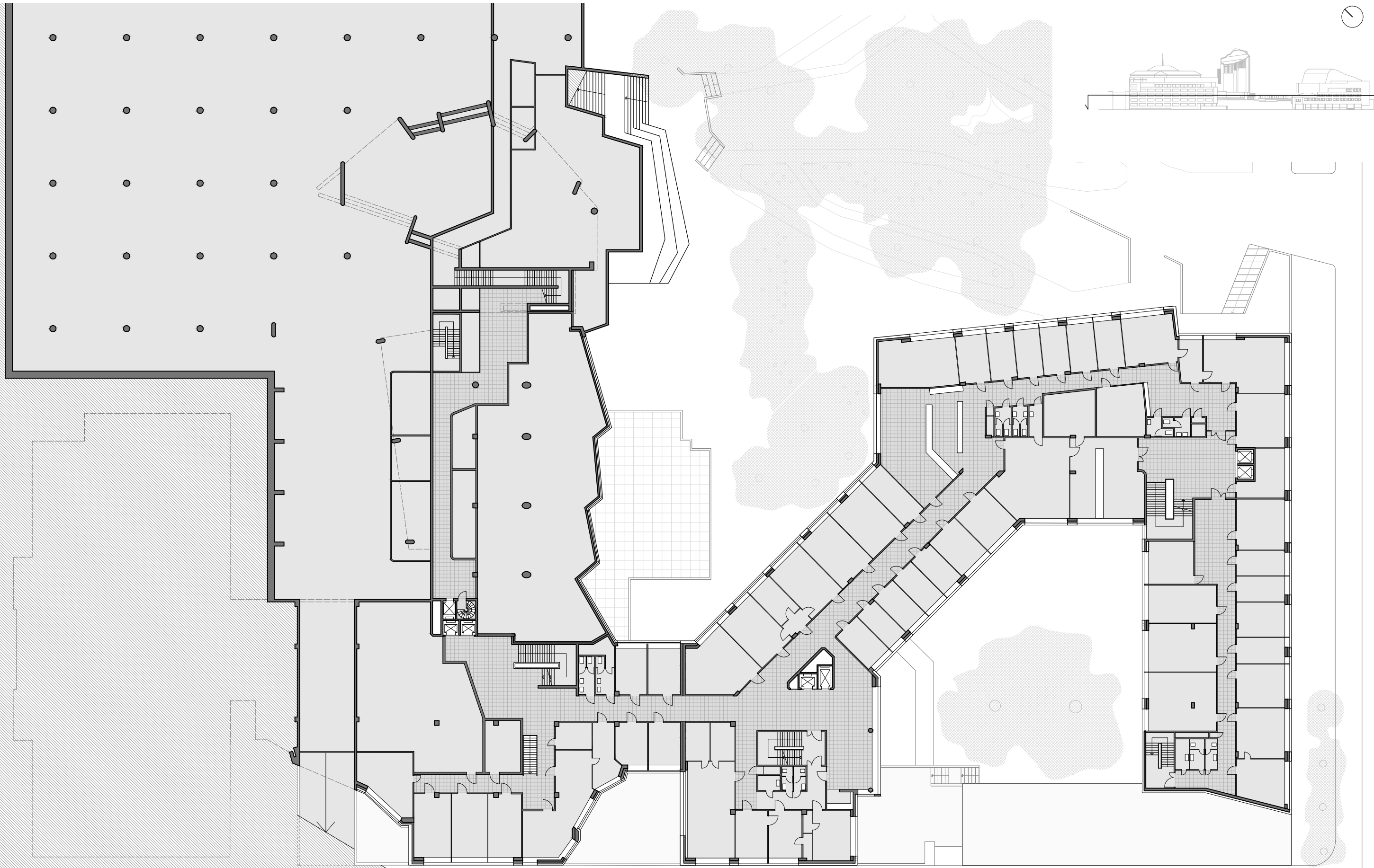
Planta inferior
