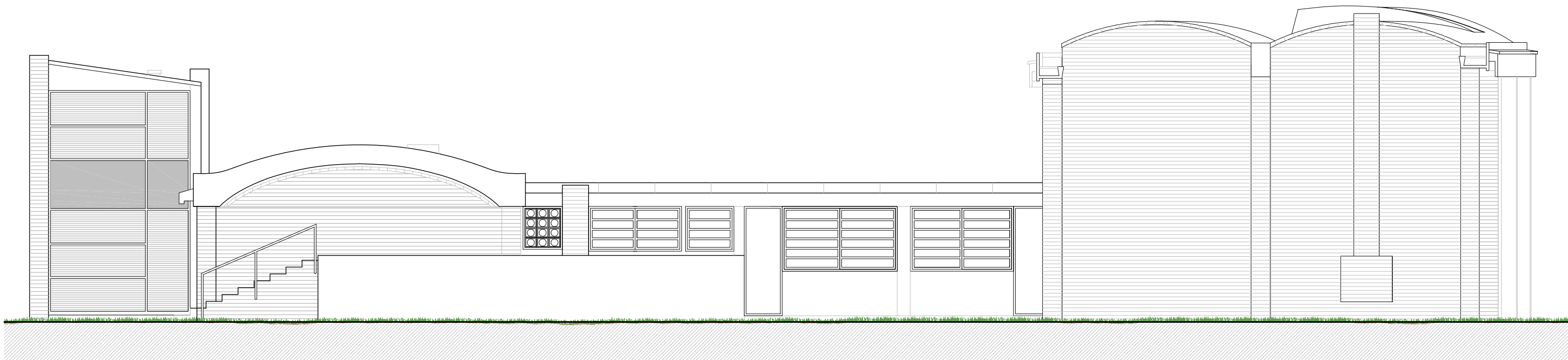
Seccions d-d'
