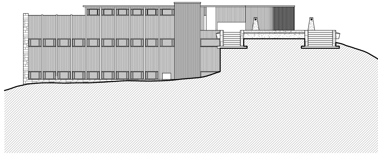
Alçat Nord-Oest
