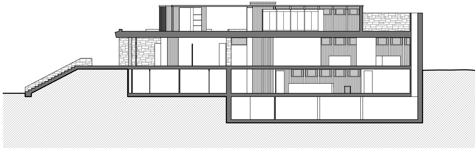
Secció transversal
