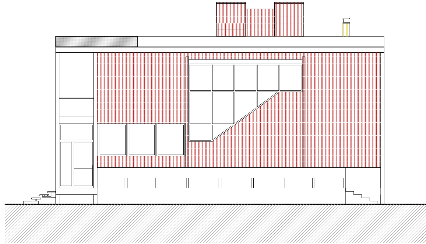
Alçat Oest
