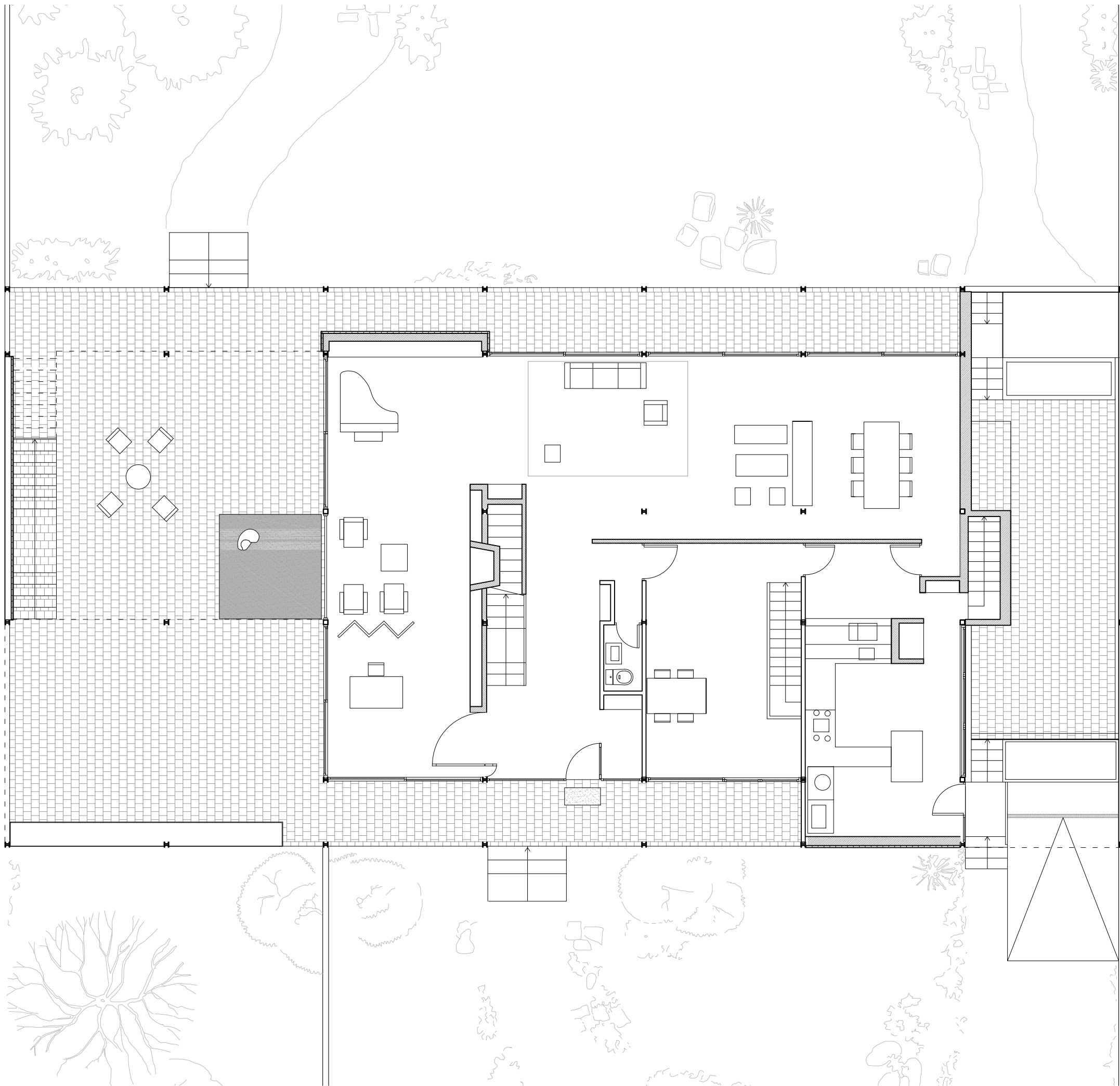
Planta Baixa
