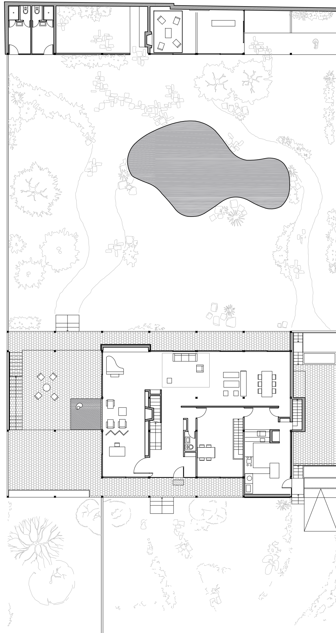
Planta parcel·la
