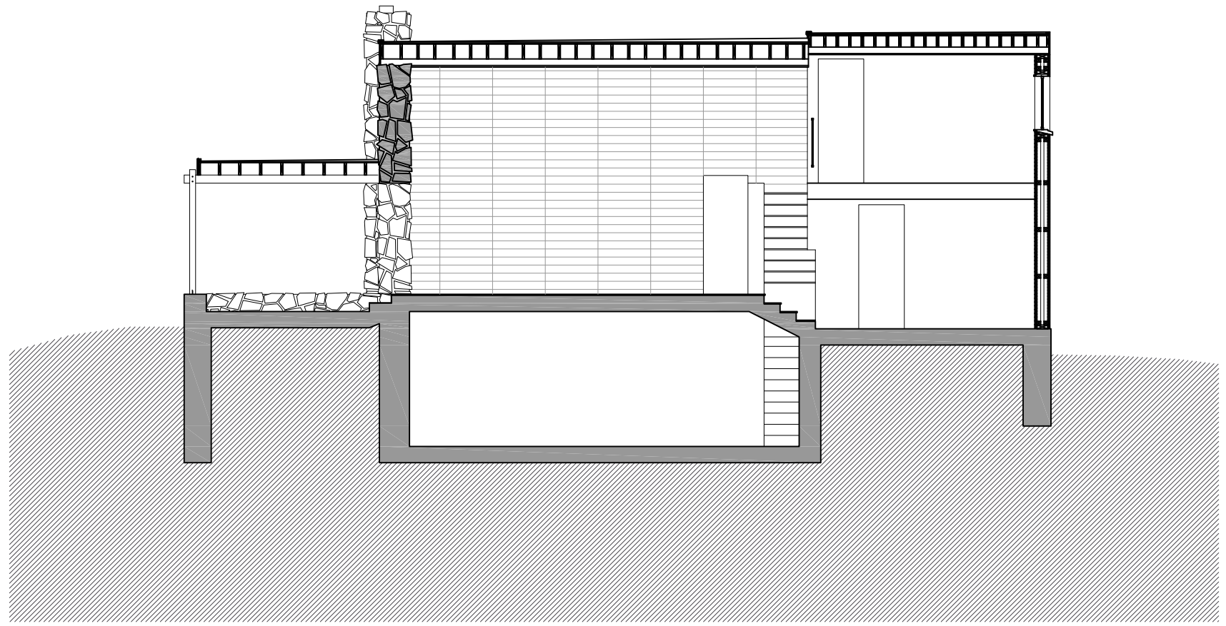
Secció longitudinal
