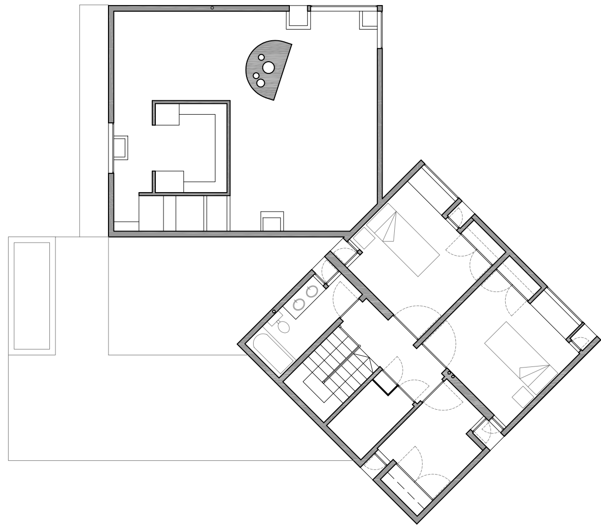
Planta Primera
