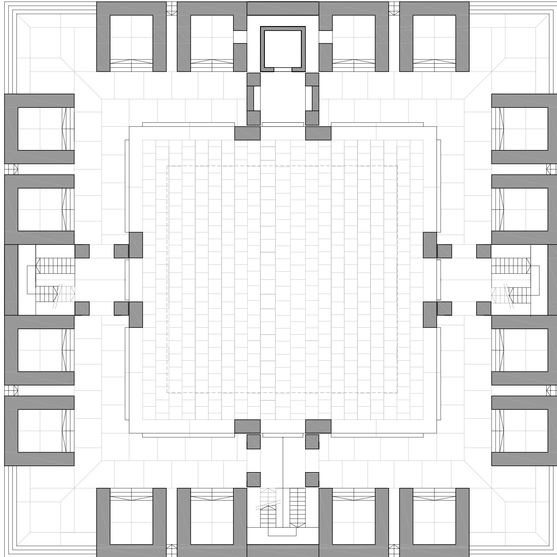
Planta Baixa
