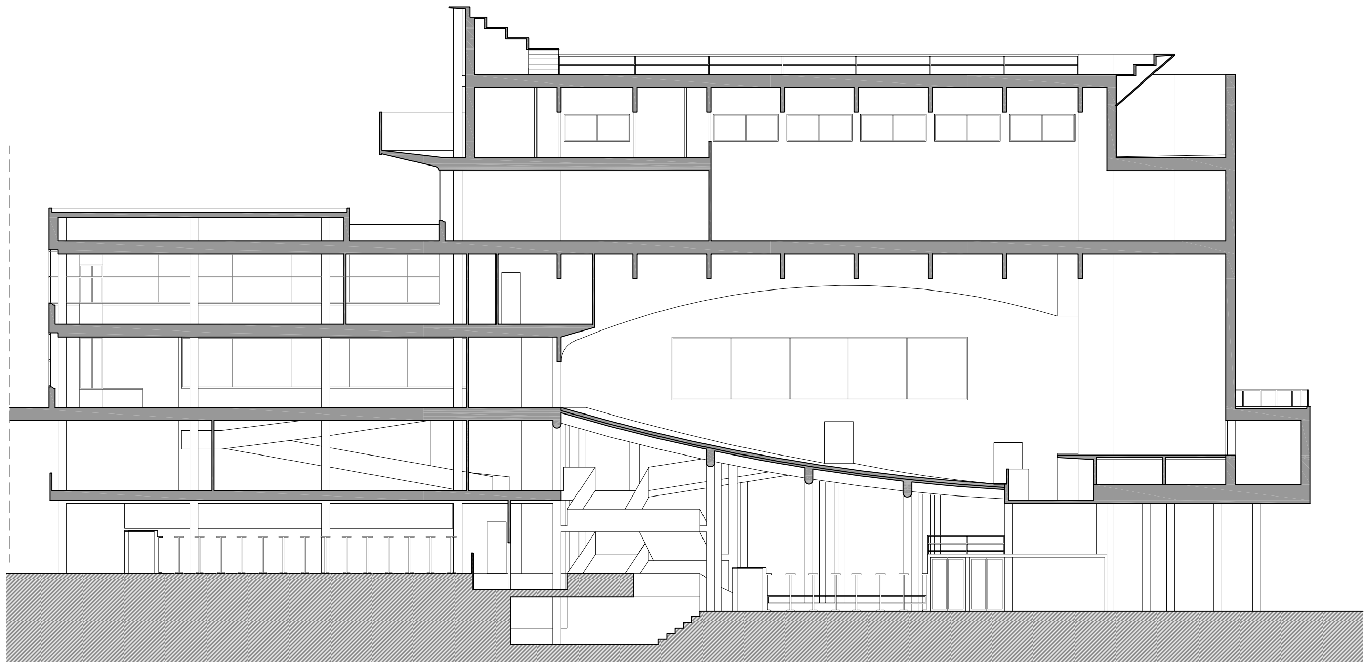
Alçat secció h-h'
