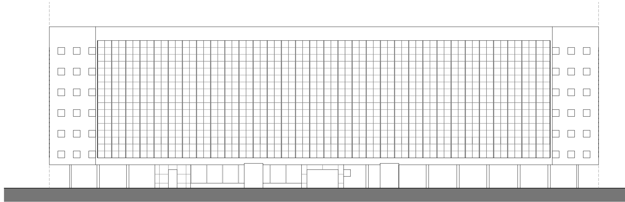
Alçat general sobre la Miasnitzkaia (a-a')
