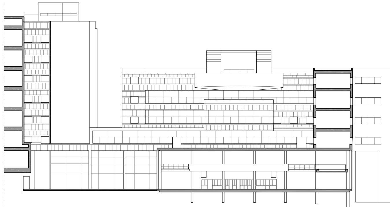
Alçat secció g-g'
