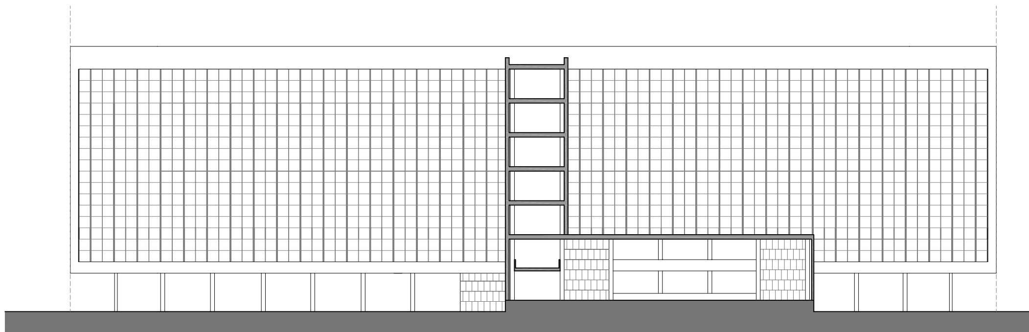
Alçat-secció b-b'
