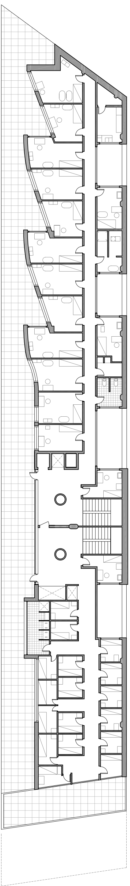
Planta 6
