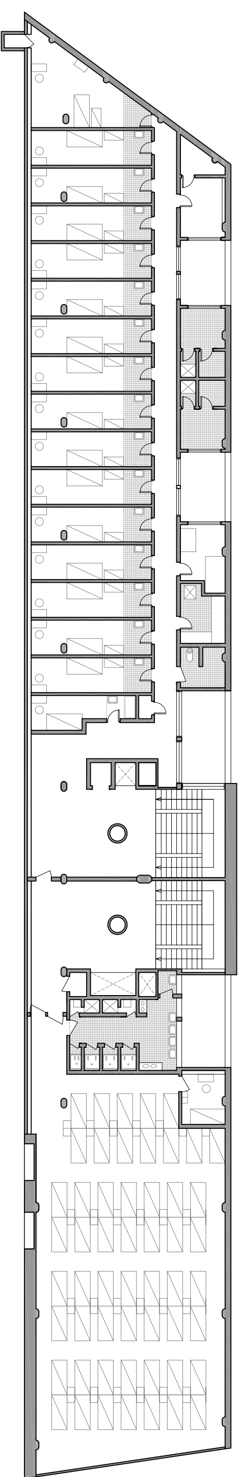
Planta Tipus
