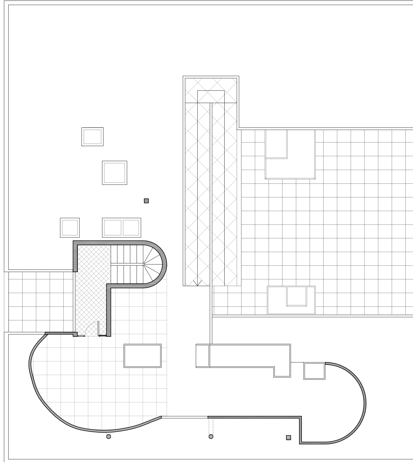
Planta Cobertes
