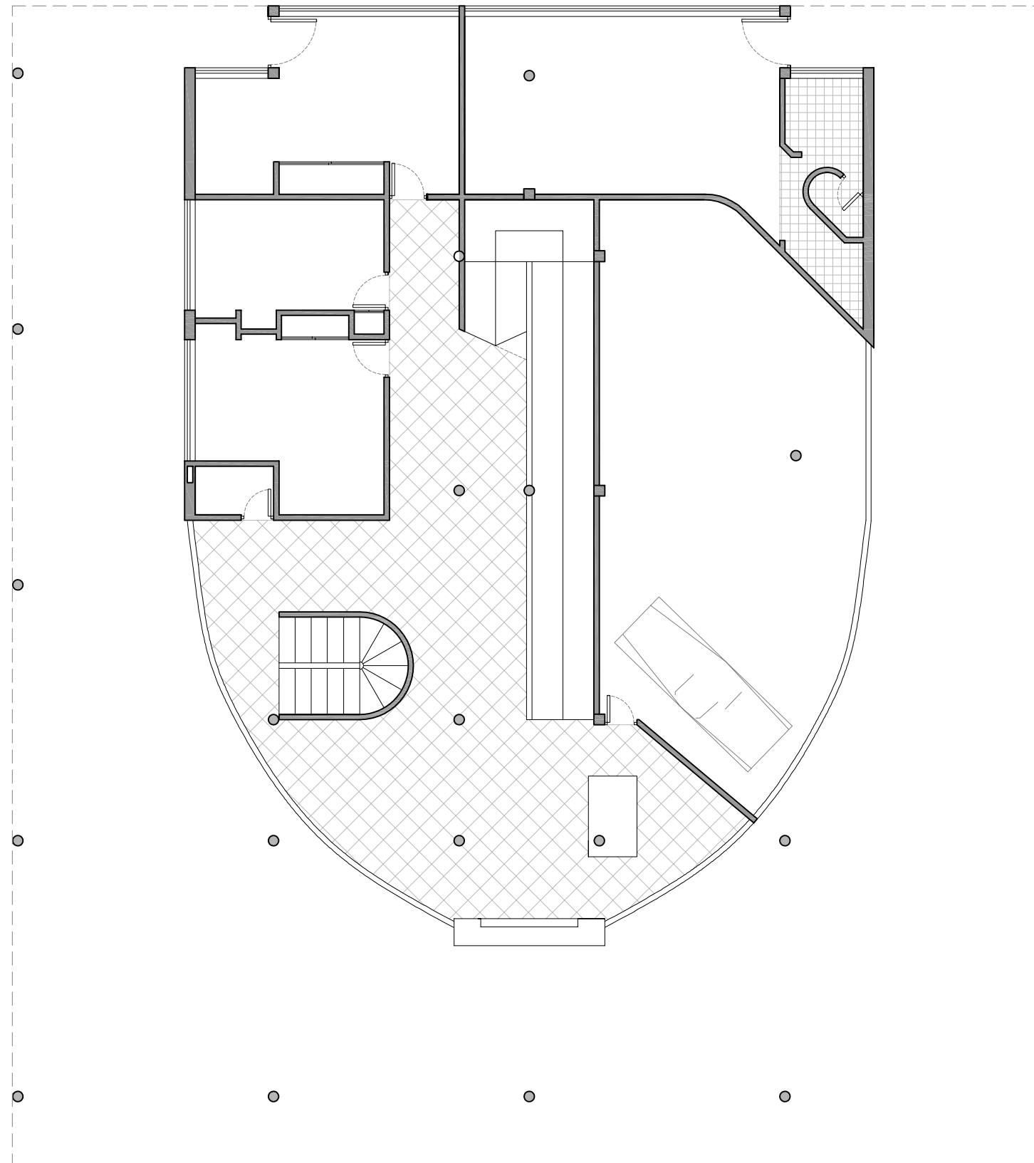
Planta Baixa
