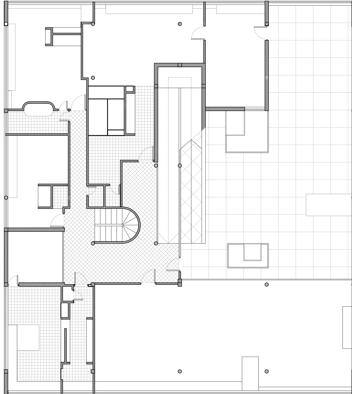
Planta Primera
