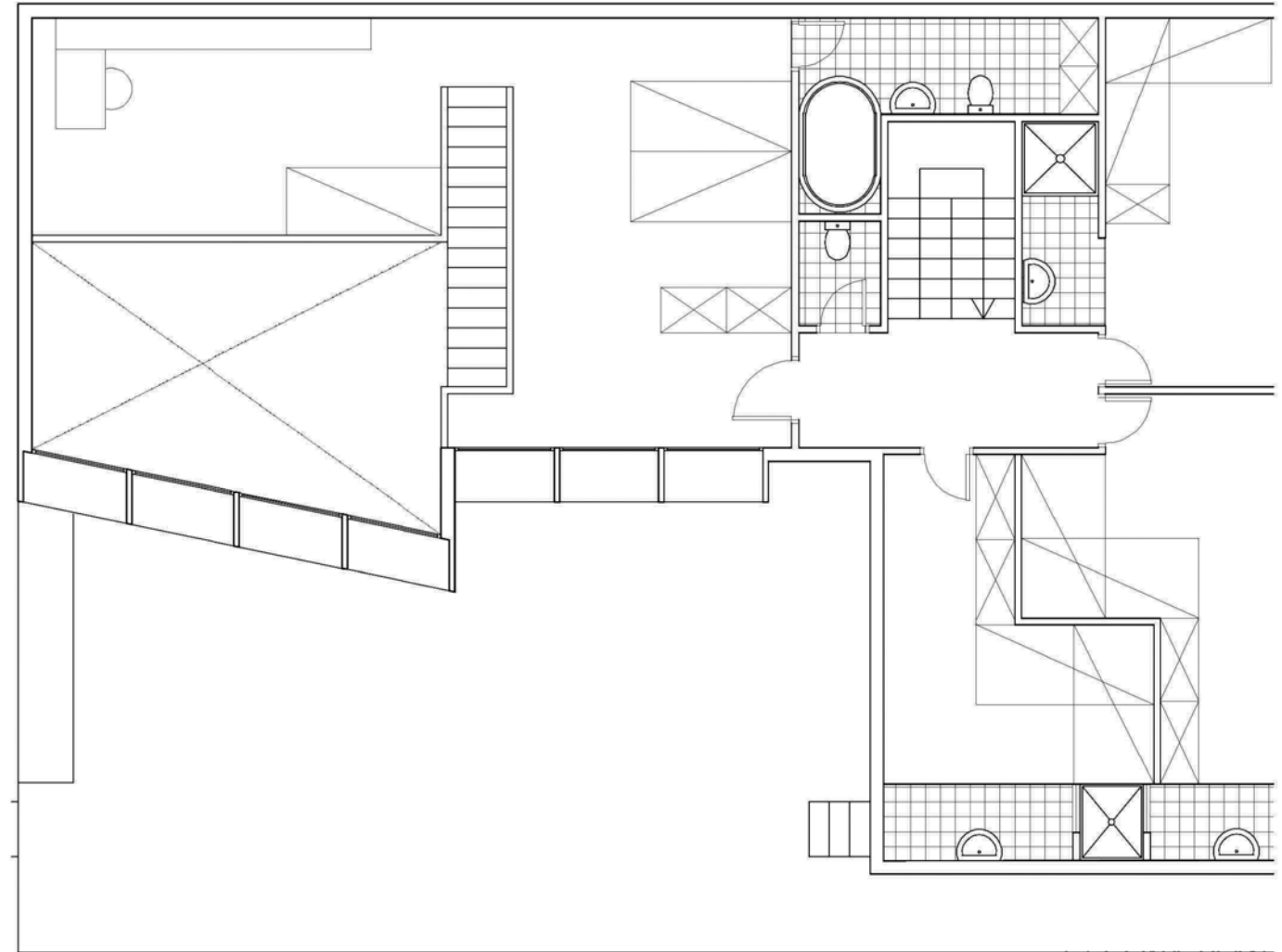
segona planta
