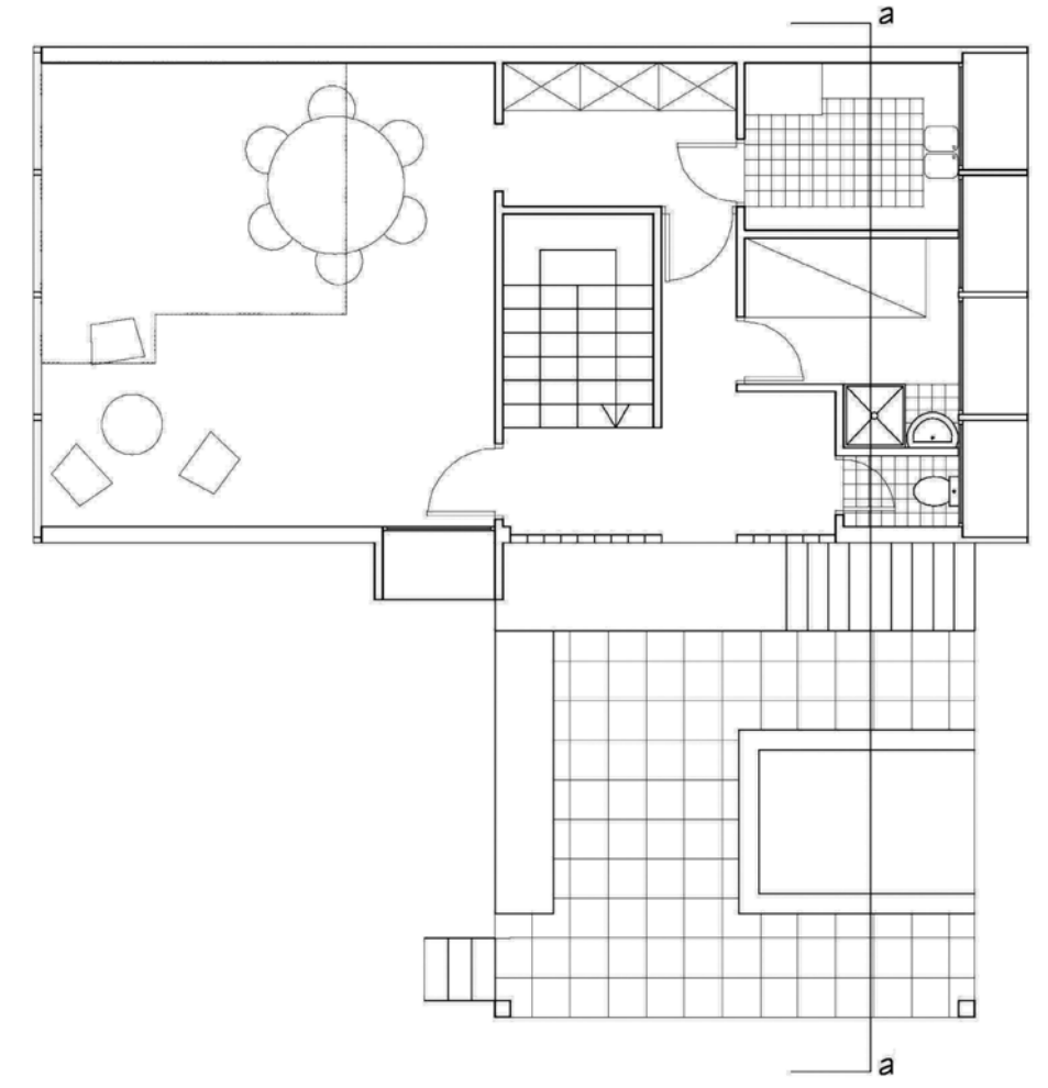
primera planta
