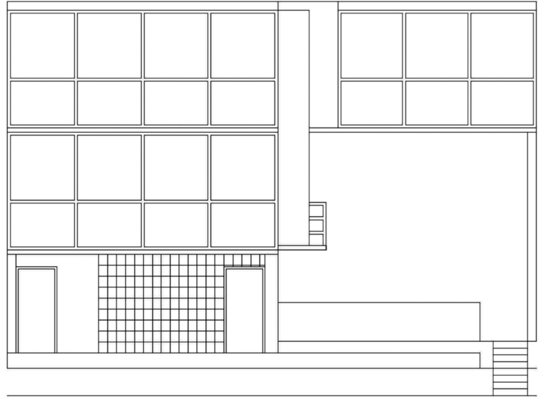
Façana nord-est
