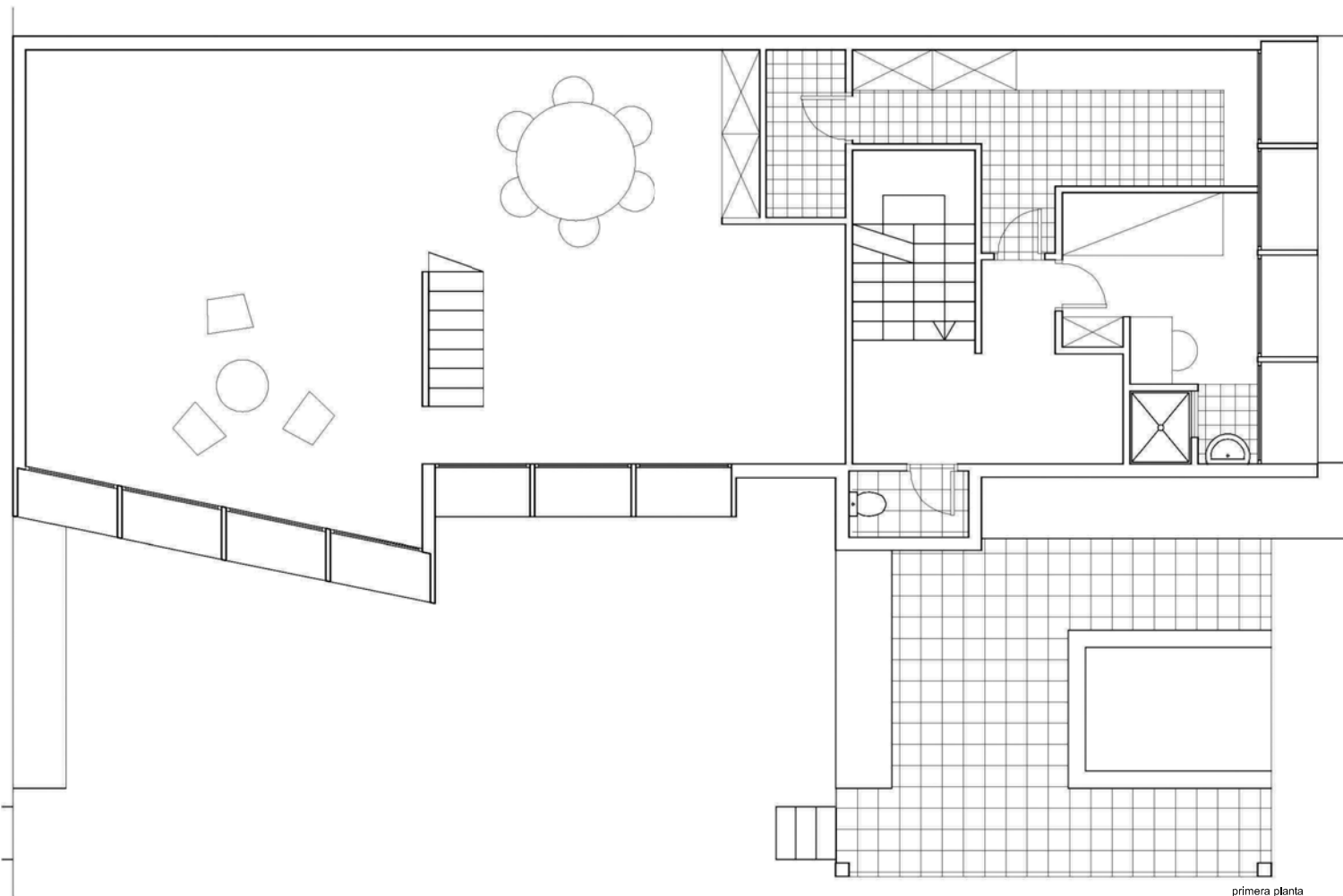
primera planta
