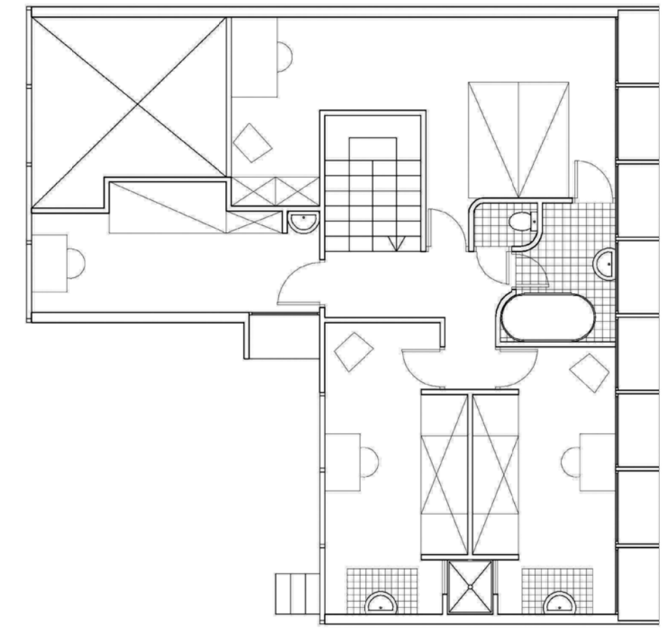
segona planta
