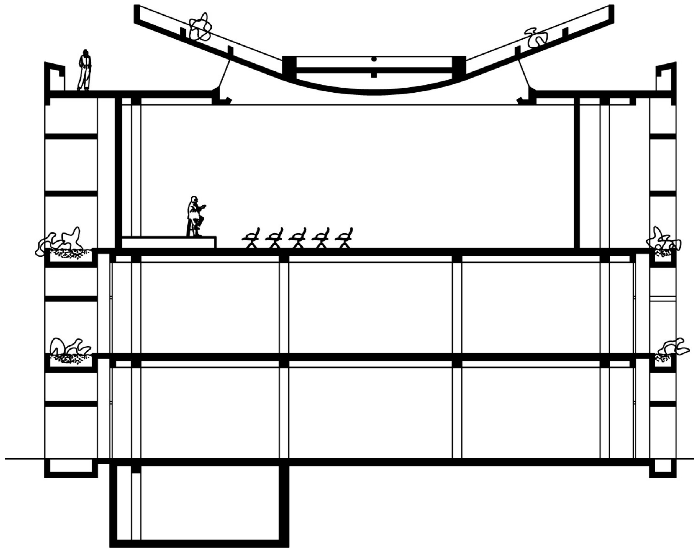
Secció Longitudinal
