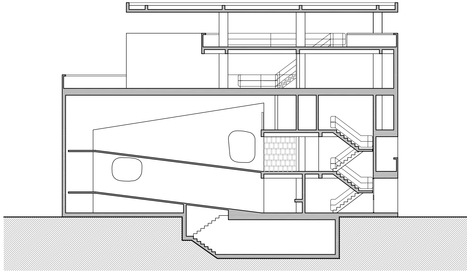
Secció Longitudinal
