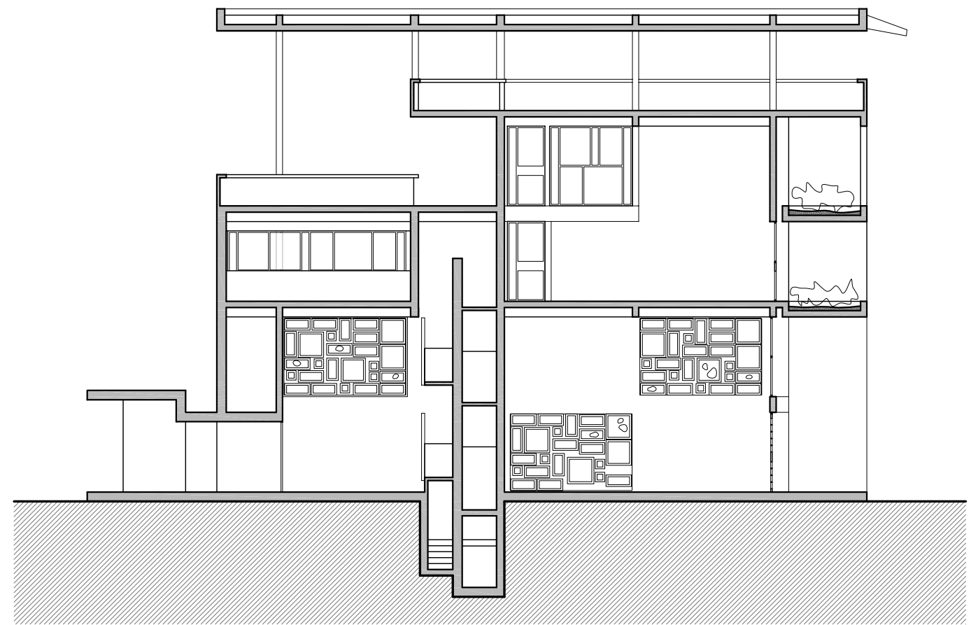
Secció Transversal
