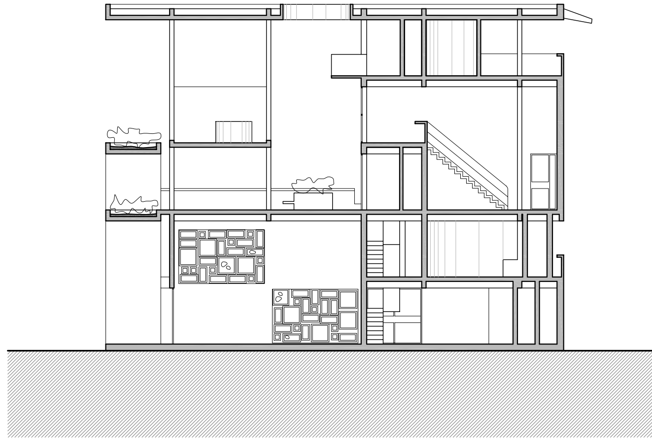
Secció Transversal
