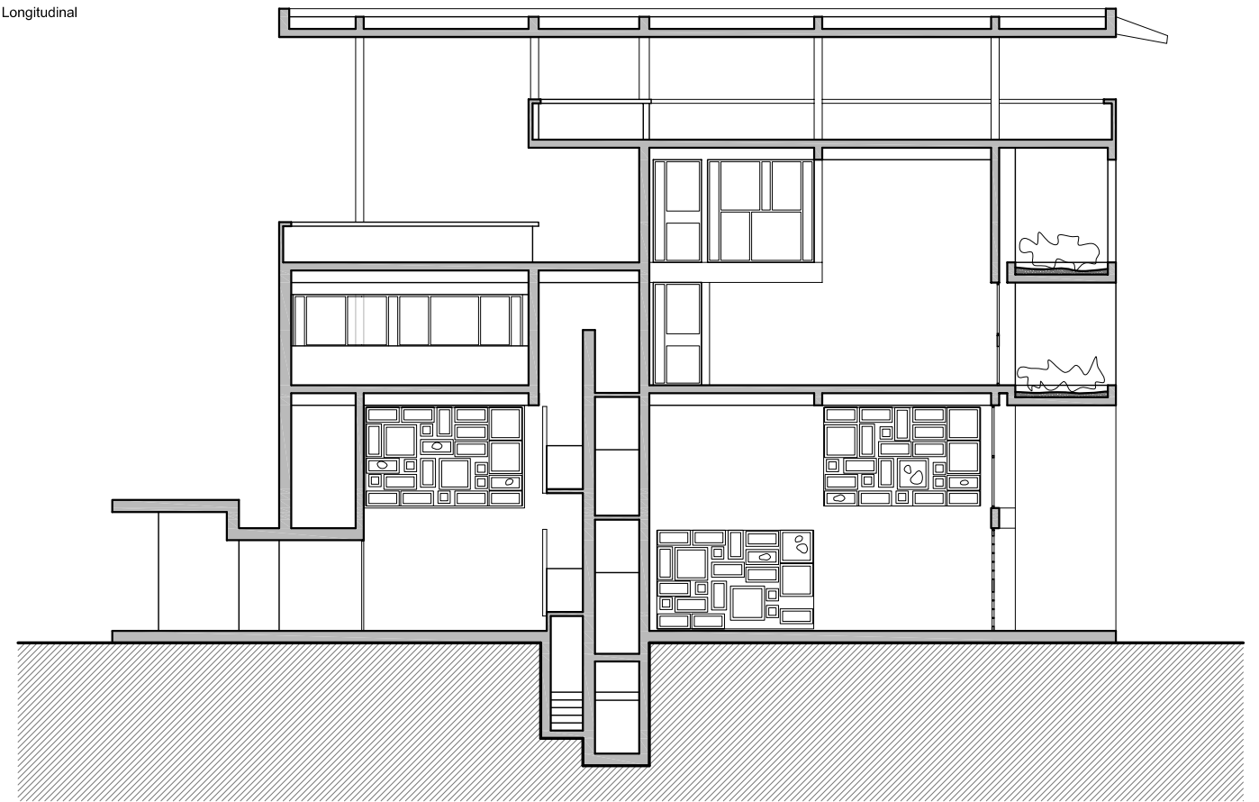
Secció Longitudinal
