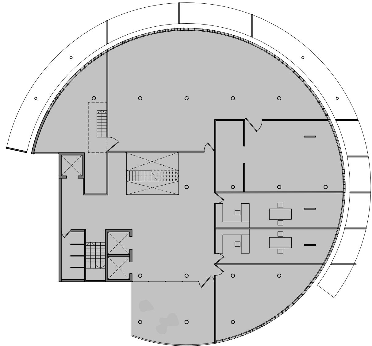
Planta Cinquena
