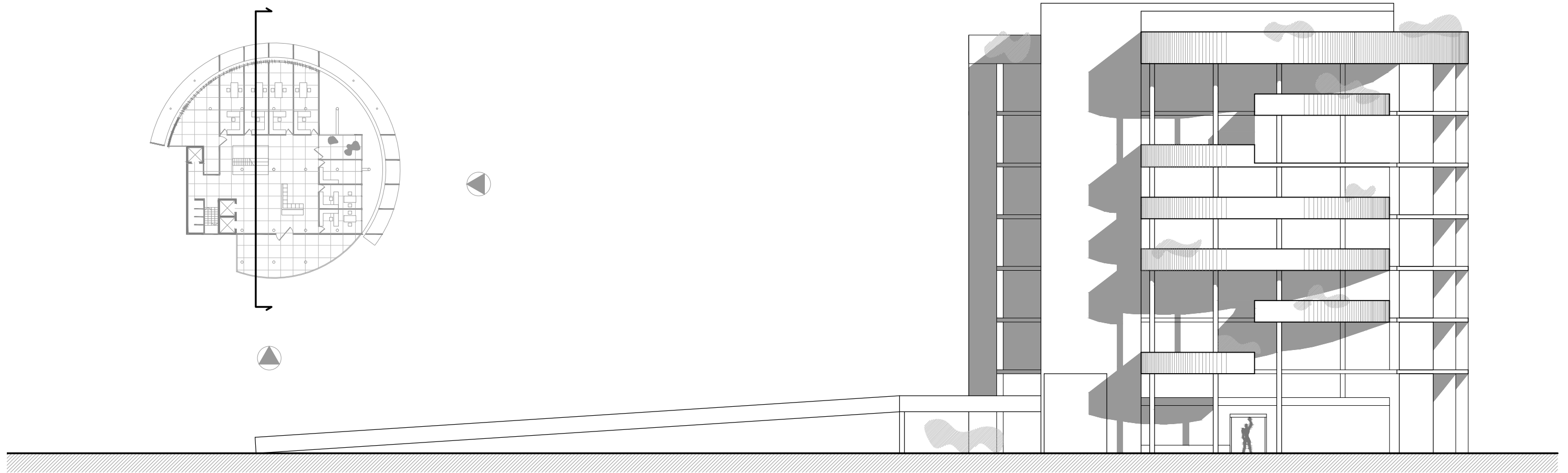
Alçat Sud-est
