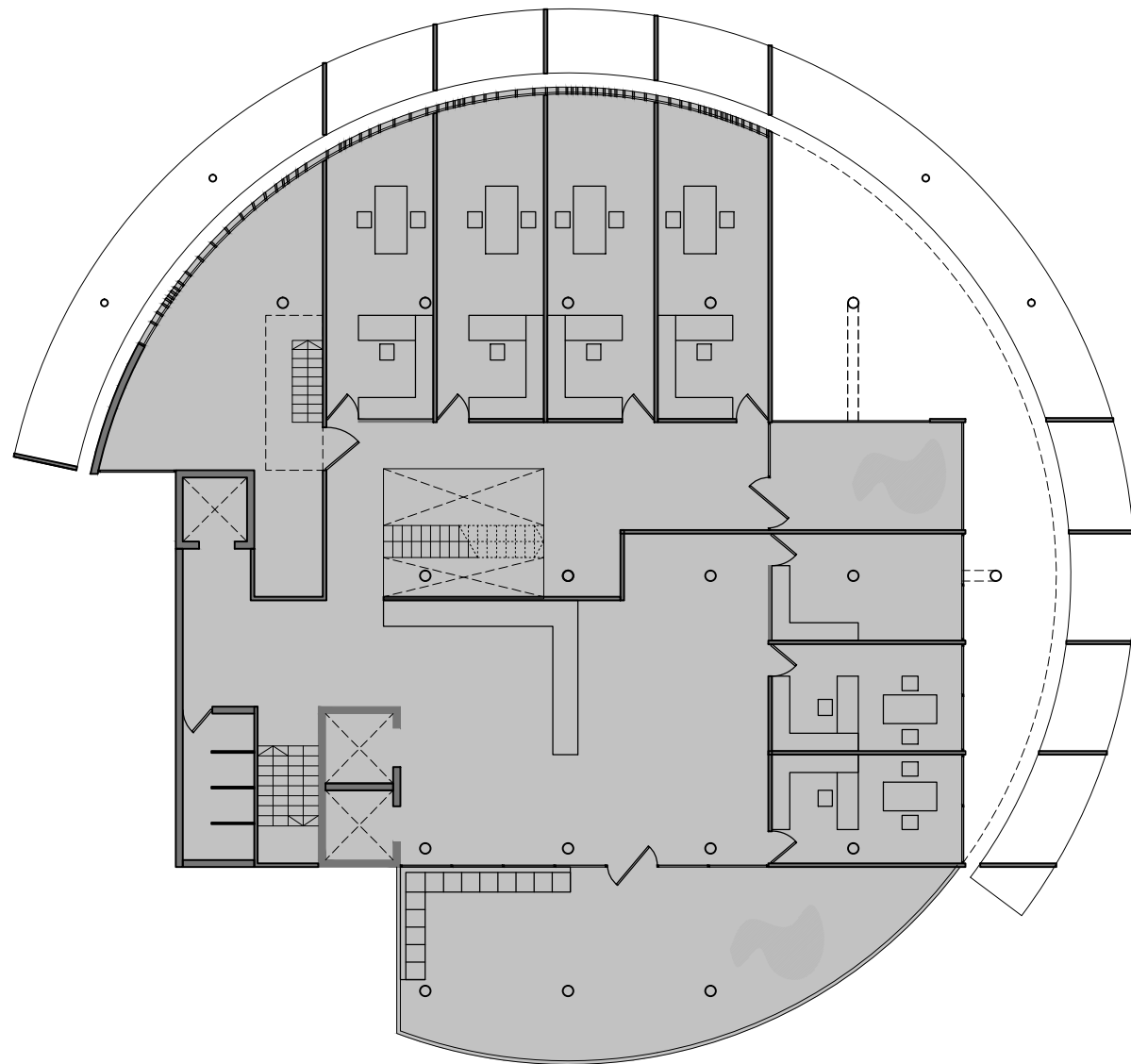
Planta Quarta
