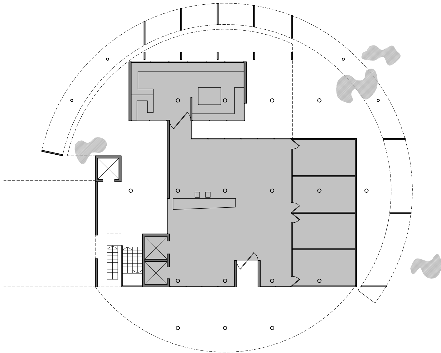
Planta Baixa
