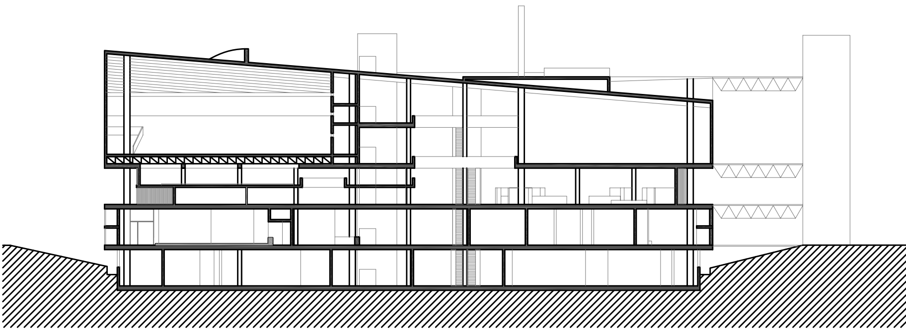
Seccion A-A'
