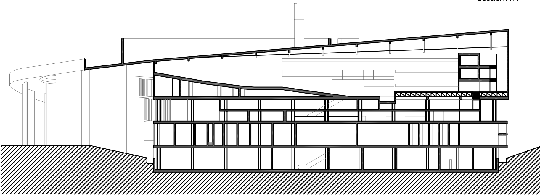
Seccion B-B'
