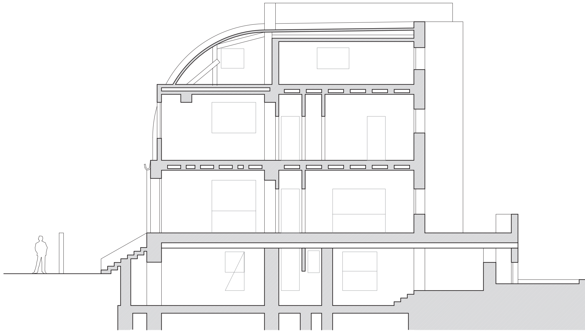
Secció Transversal
