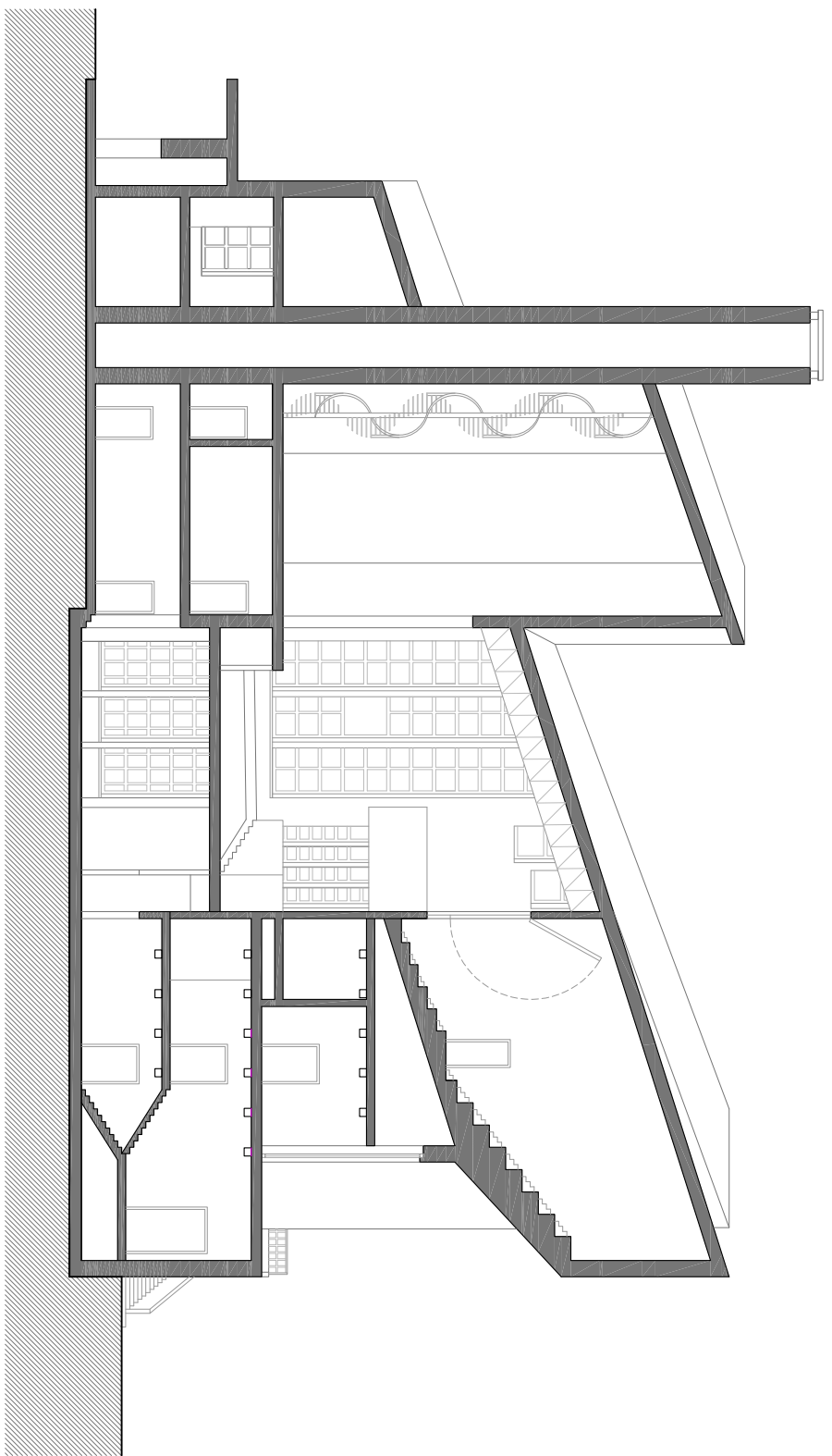
Secció longitudinal
