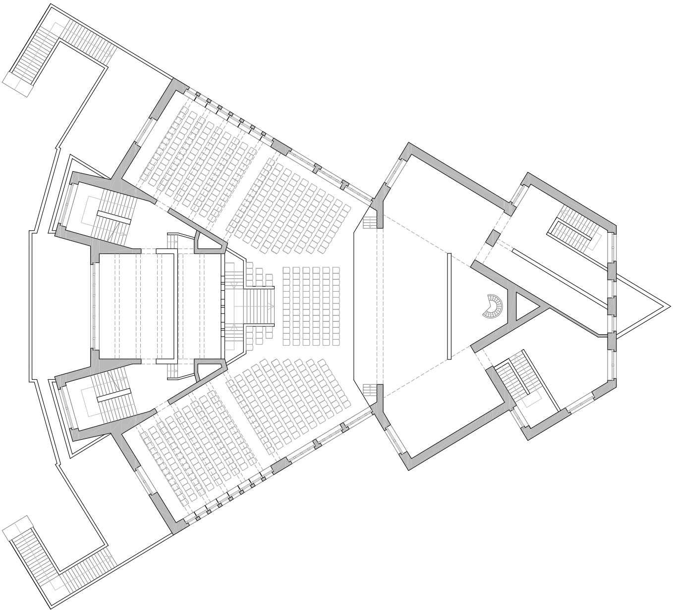
Planta segunda
