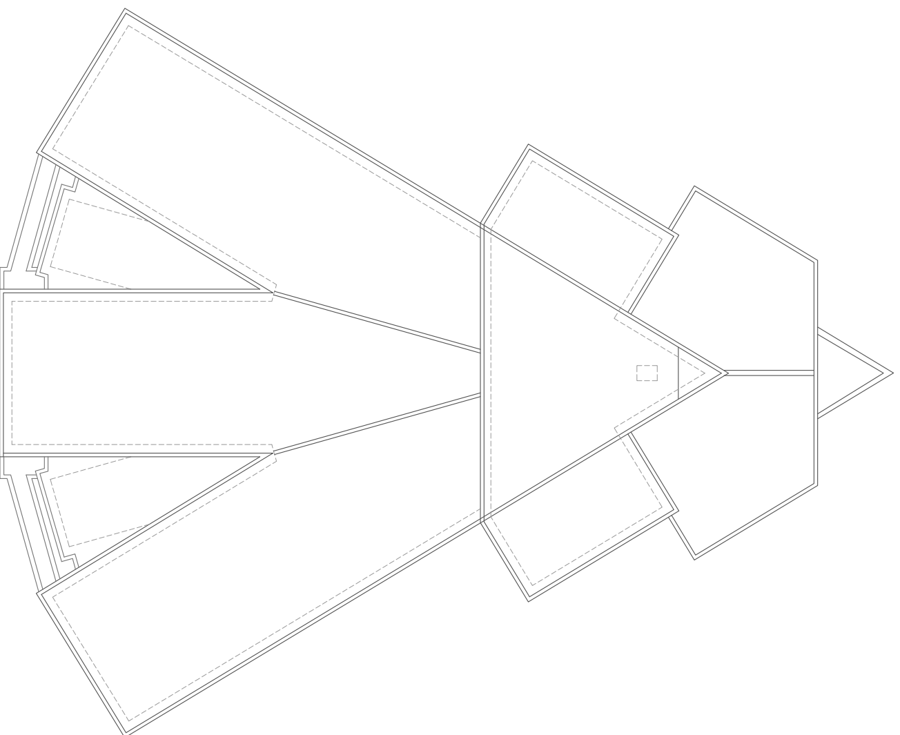
Planta de coberta
