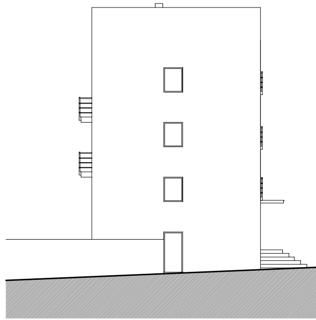
Alçat Nord
