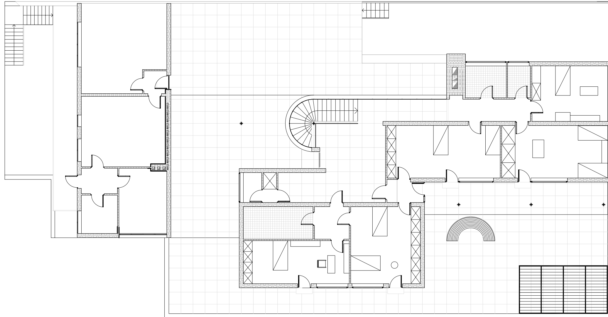
Planta Primera
