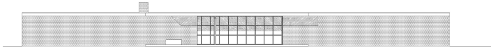
Alçat sud-est
