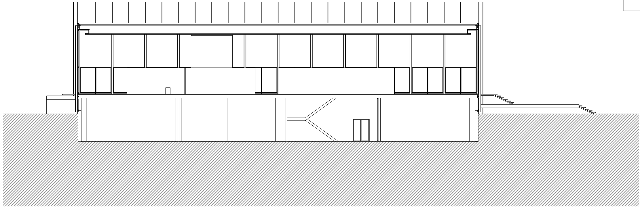
Secció A-A'
