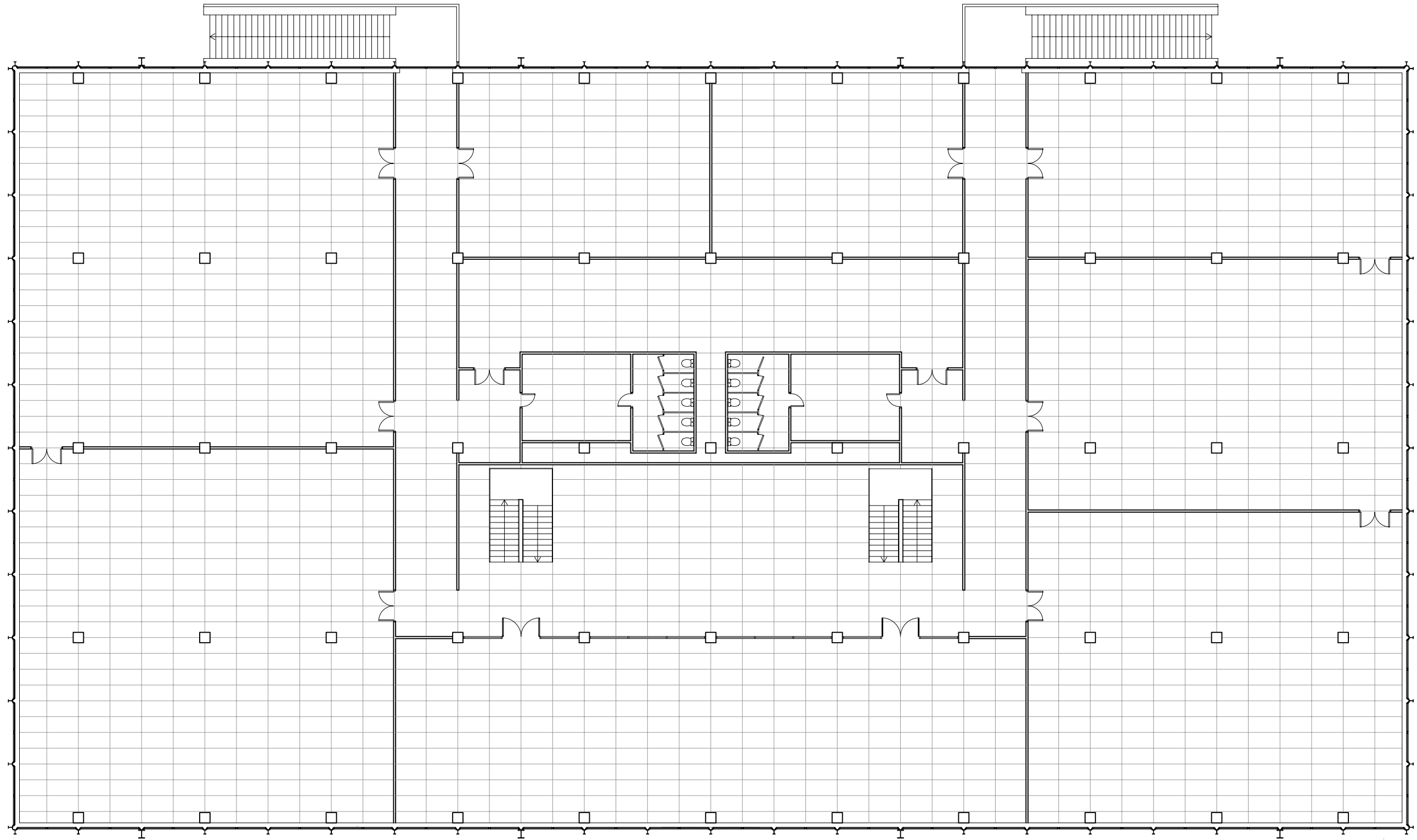
Planta Soterrani
