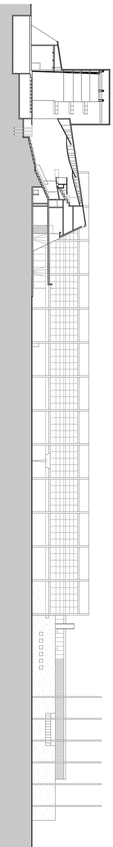
Secció DD
