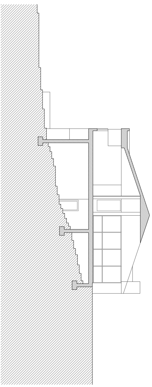
Secció DD
