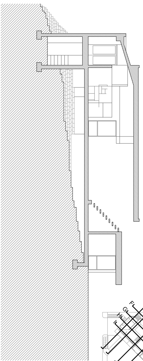
Secció GG
