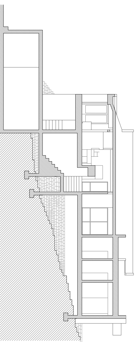
Secció II
