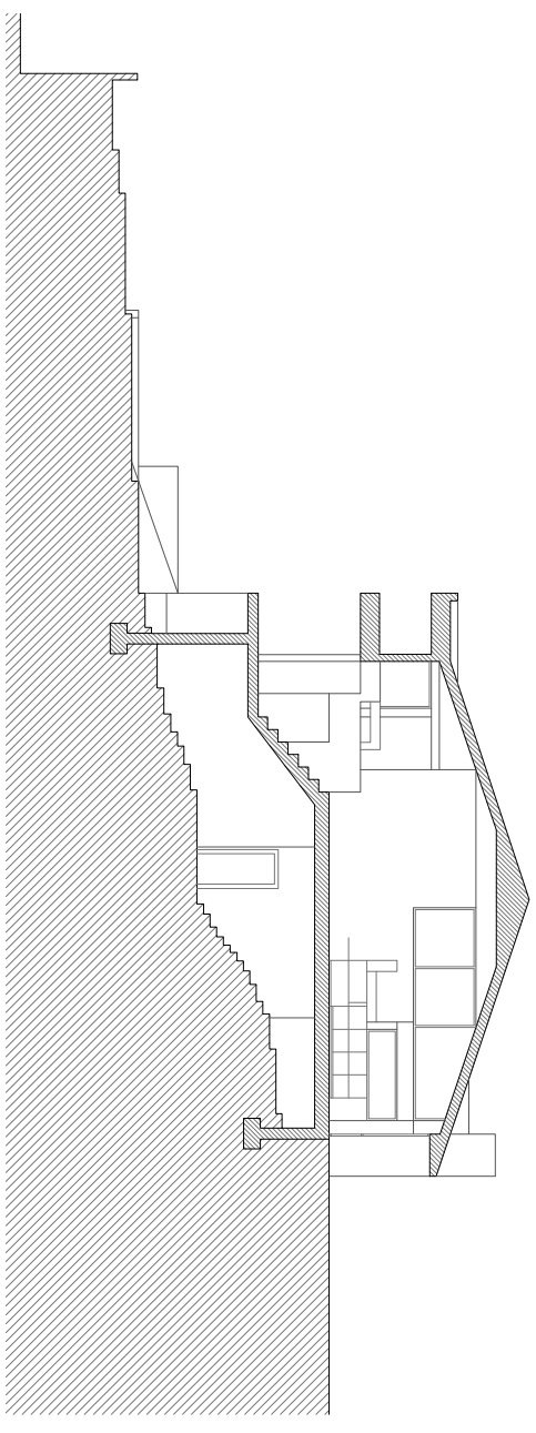
Secció CC
