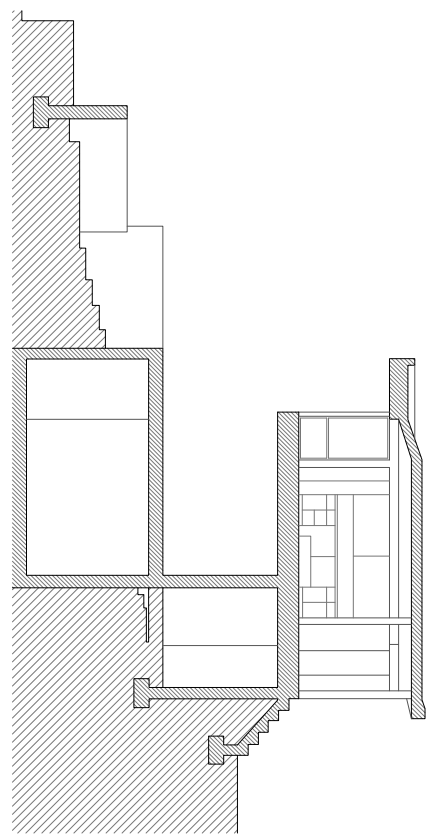
Secció AA
