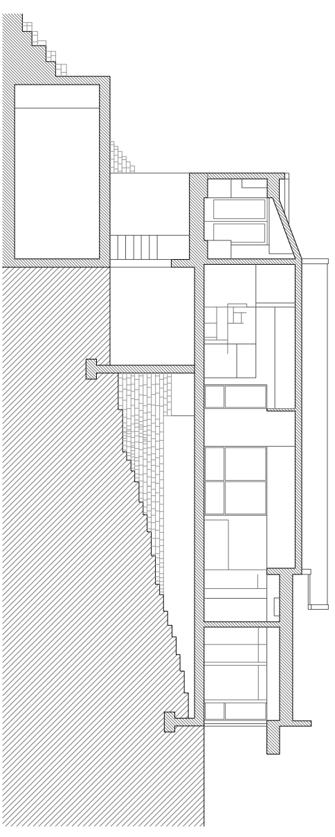
Secció HH
