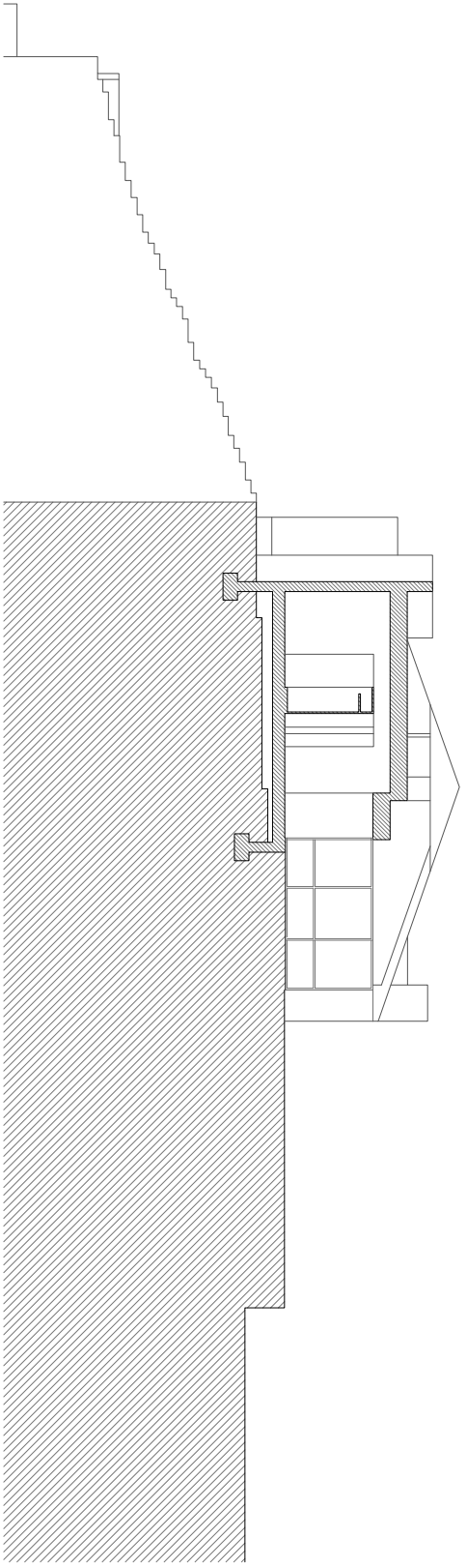
Secció EE
