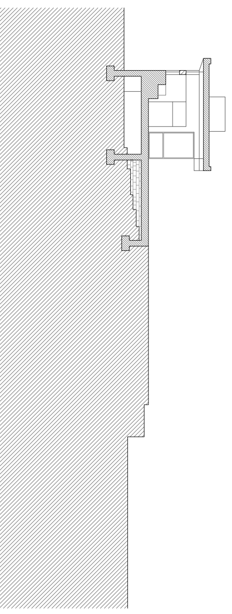
Secció FF
