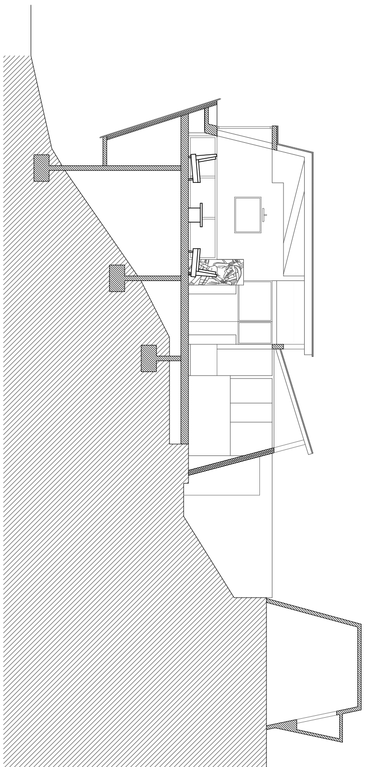
Secció CC
