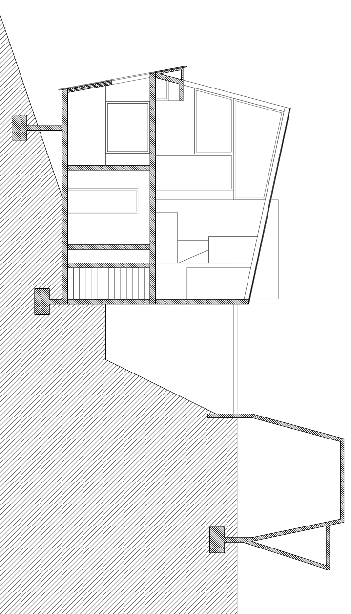
Secció DD
