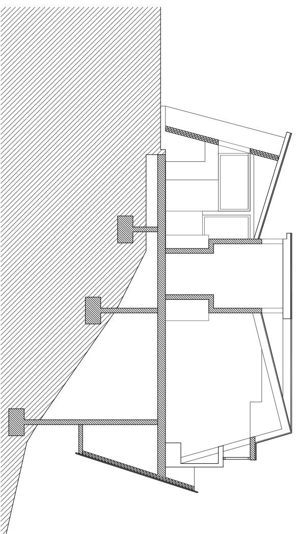
Secció AA
