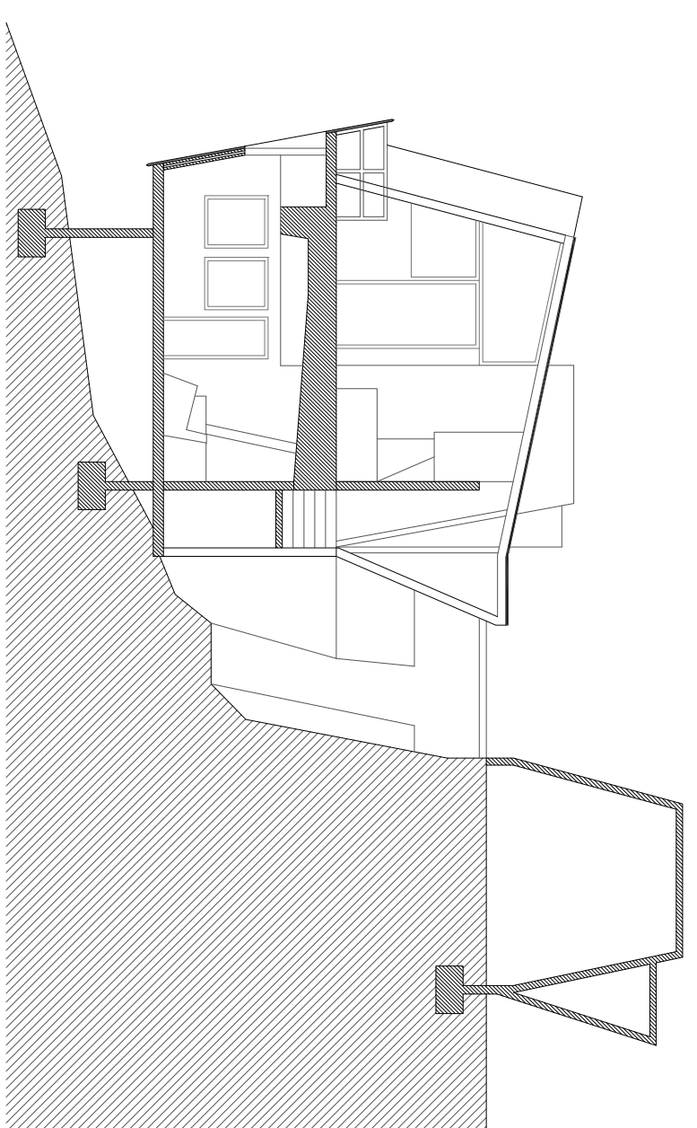
Secció EE
