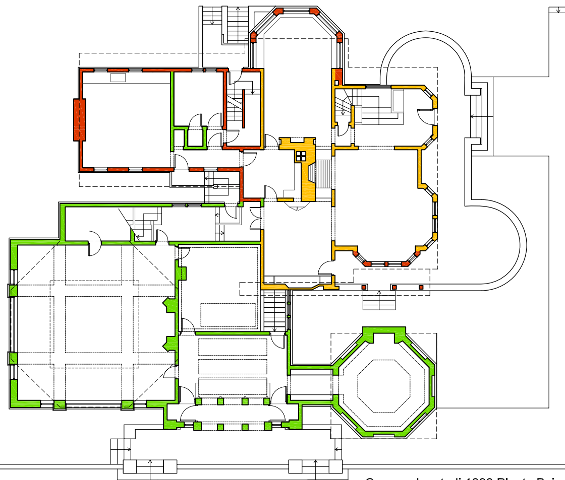
Casa amb estudi 1898 Planta Baixa
