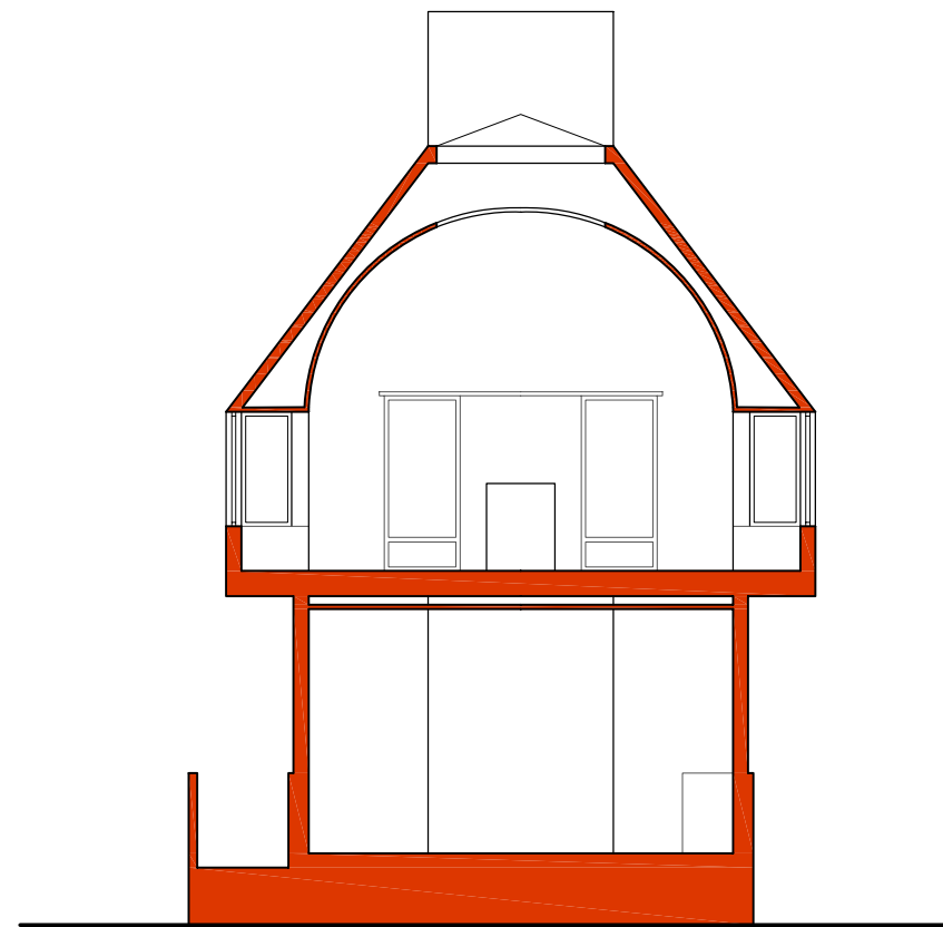
Secció Transversal T3
