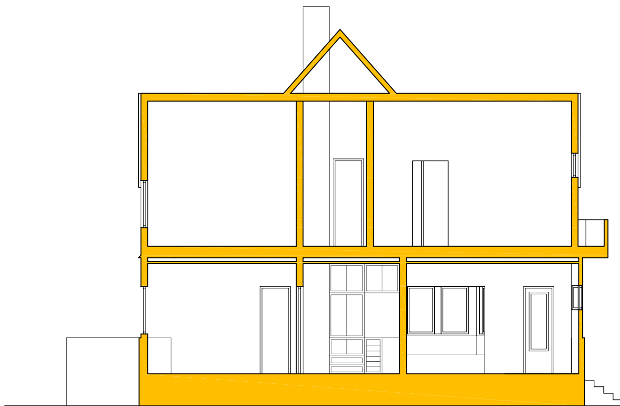
Secció Transversal T2
