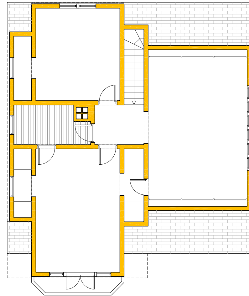
Casa 1889 - Planta Pis
