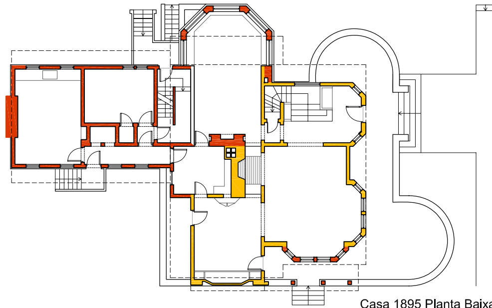
Casa 1895 Planta Baixa
