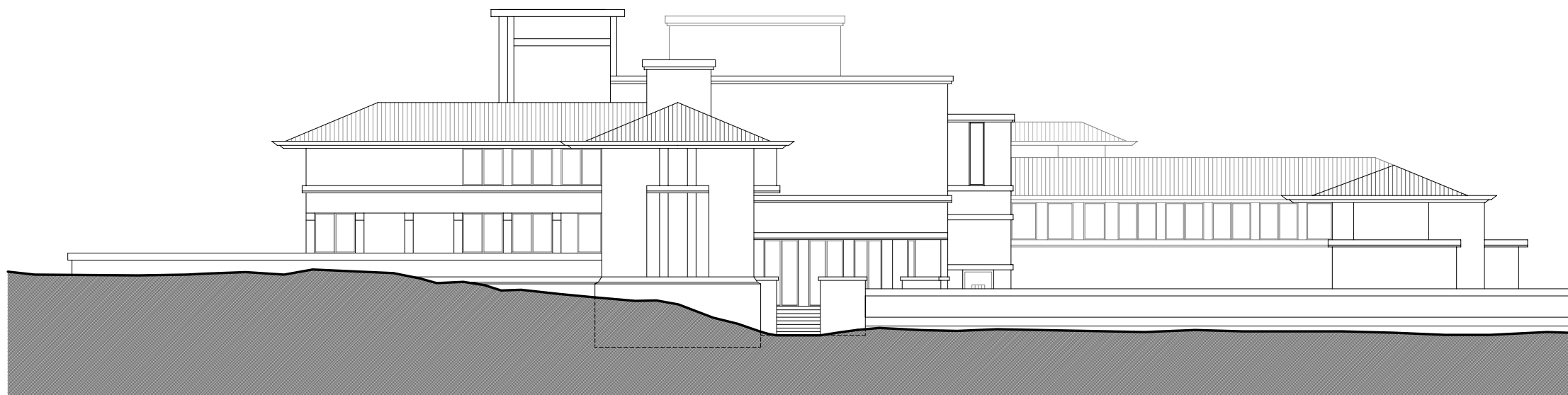
Alçat Sud
