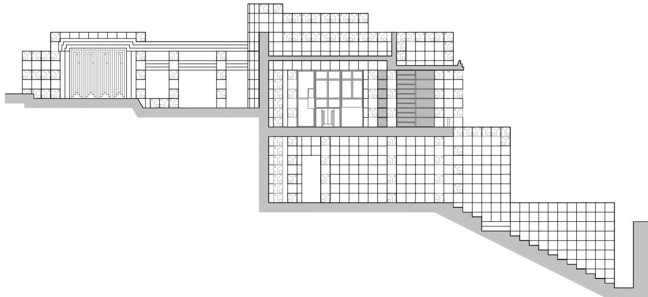
Secció A-A'
