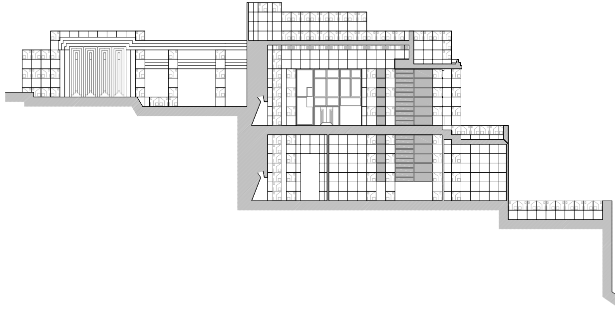
Secció B-B'
