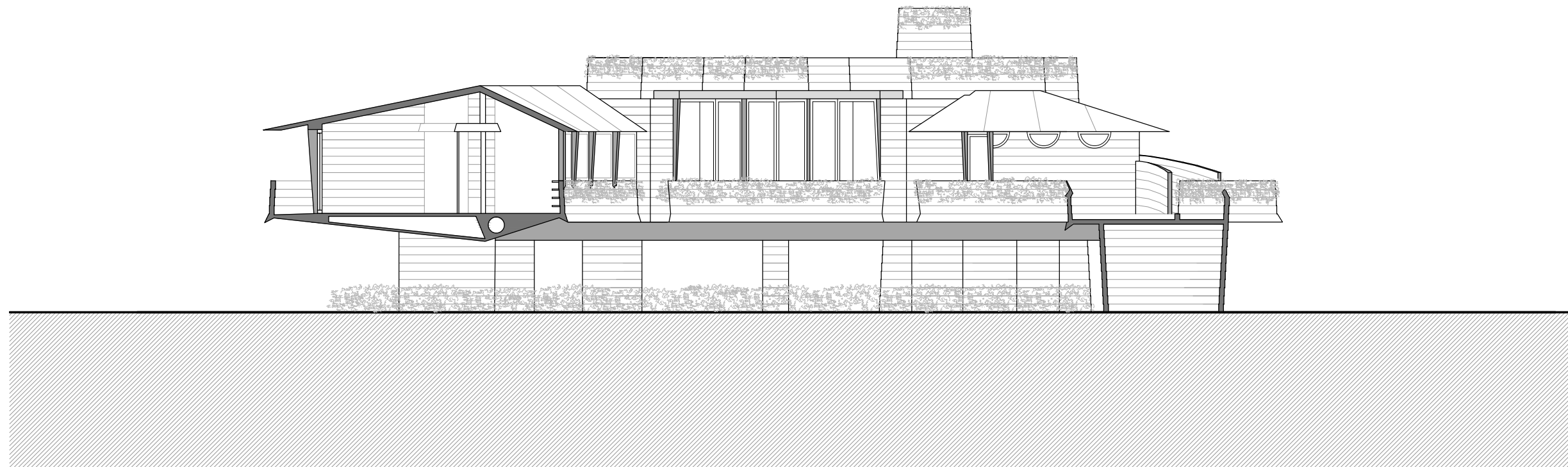
Secció a-a'
